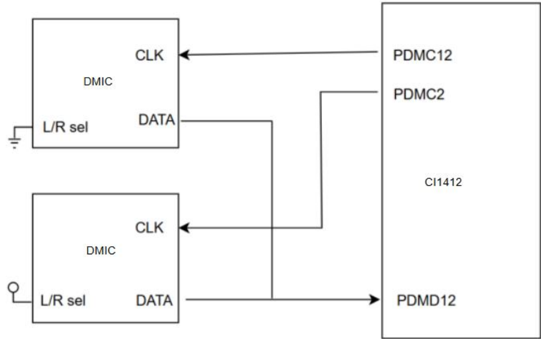
图 3：可关闭时钟连接方式
