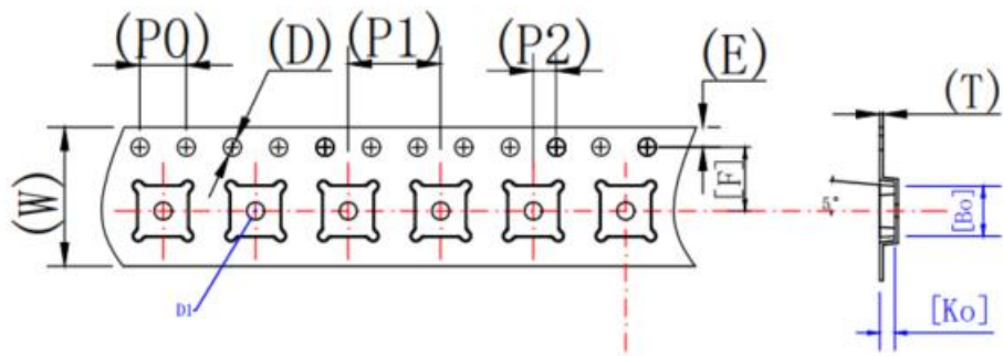
图 13：卷带尺寸图
