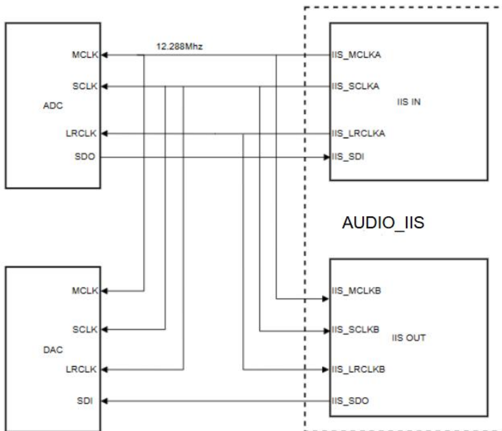
图 11：五线主模式，IIS_in 使用主模式，IIS_out 使用从模式
