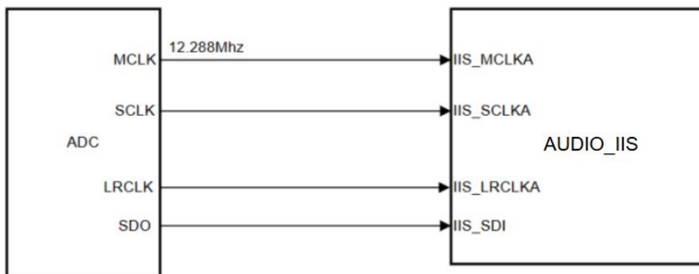
图 8:IIS 输入从模式
