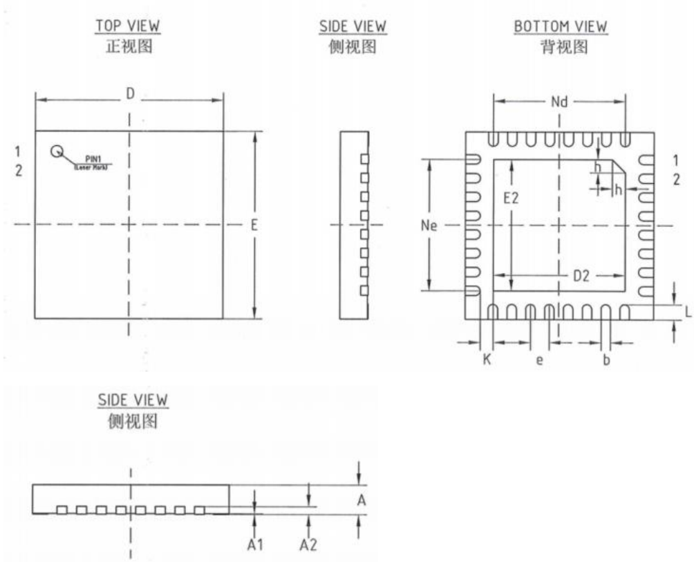
图 12: QFN32 封装尺寸
