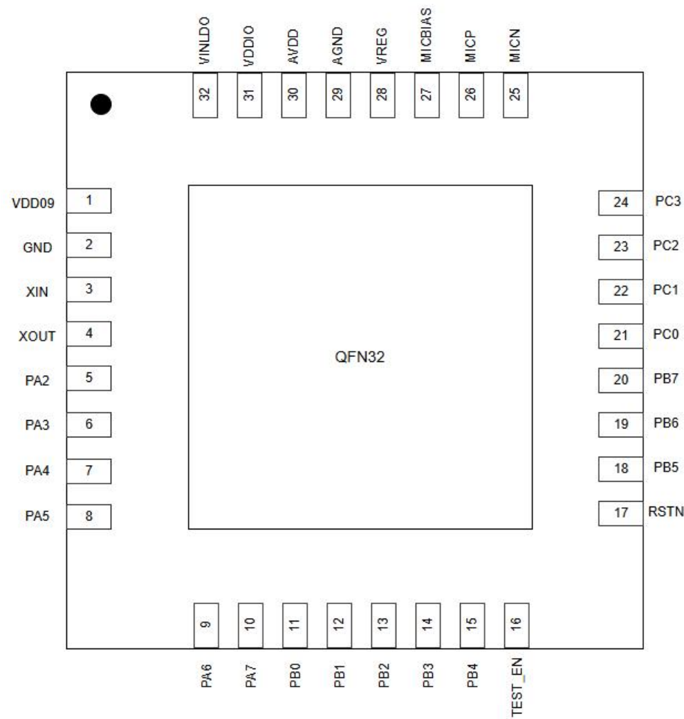
图 2：引脚图
