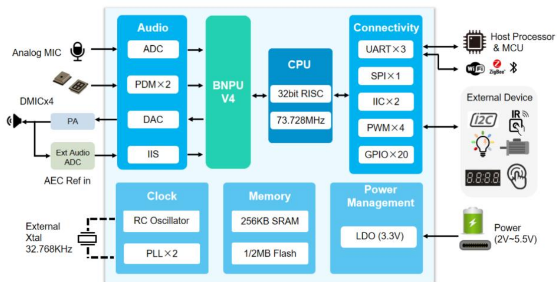
图 1：系统架构图
