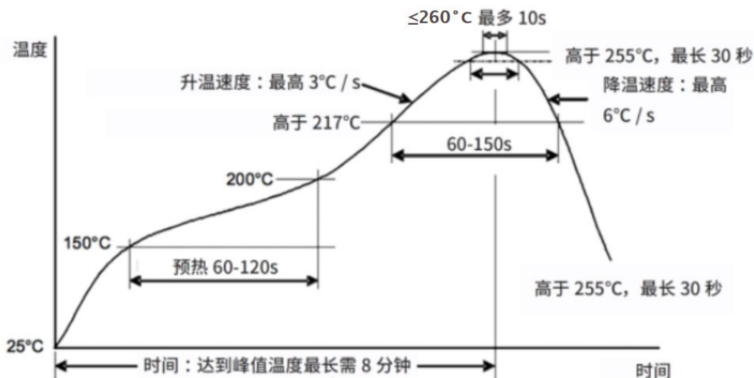
图 15: 炉温曲线图
