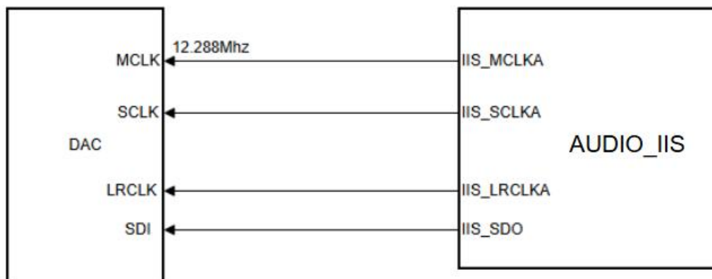
图 9: IIS 输出主模式
