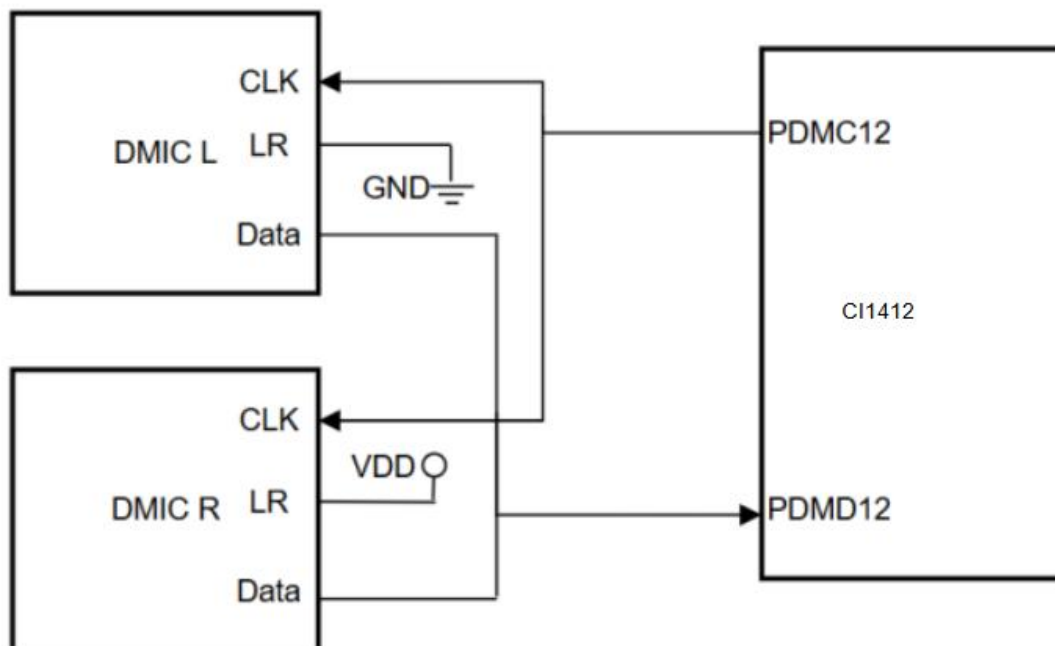
图 5: 2 路 DMIC 主模式输入
